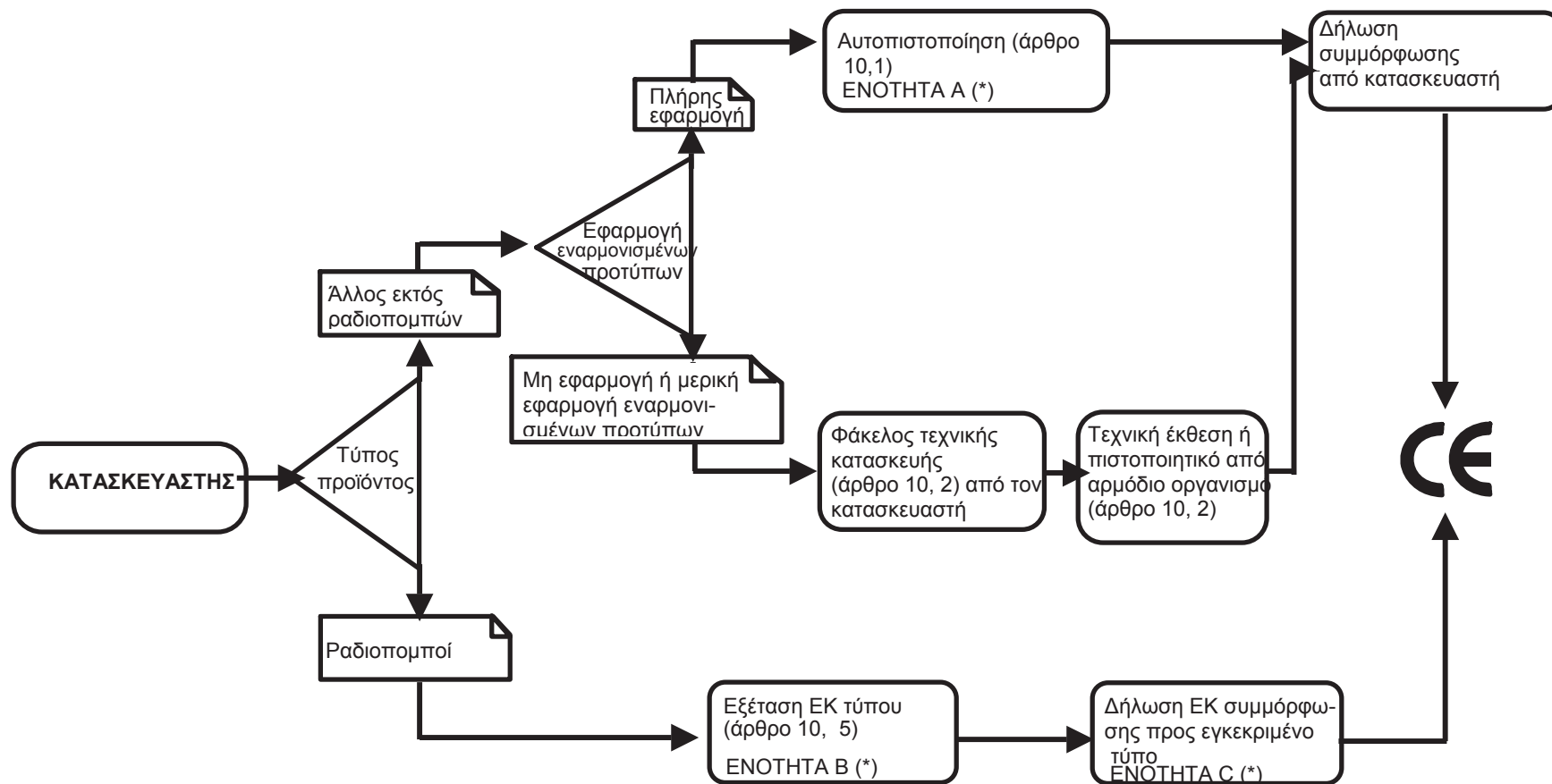
Διάγραμμα ροής για τις διαδικασίες συμμόρφωσης που προβλέπονται στην οδηγία για την ηλεκτρομαγνητική συμβατότητα
